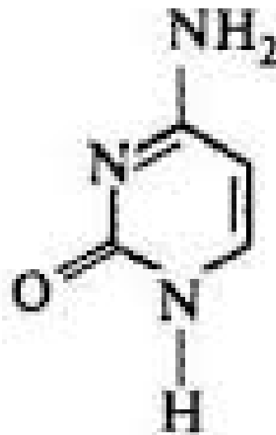
ЦИТОЗИН
